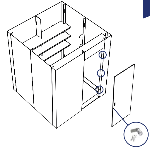
3 PORTE AMOVIBLE SERRURE A BARILLET
