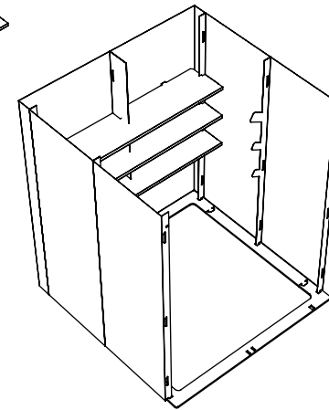
2 ASSEMBLAGE INTÉRIEUR VERROUS INVISIBLES
