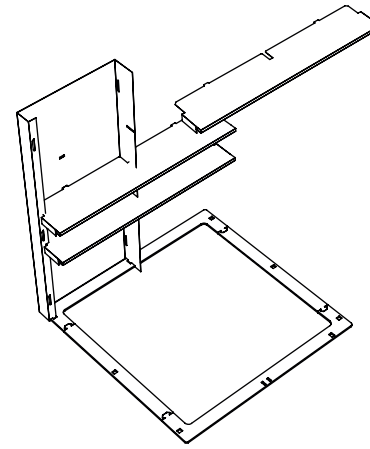
1 GUIDE AU SOL CLOISON DE FOND ET PLATEAUX DE STOCKAGE
